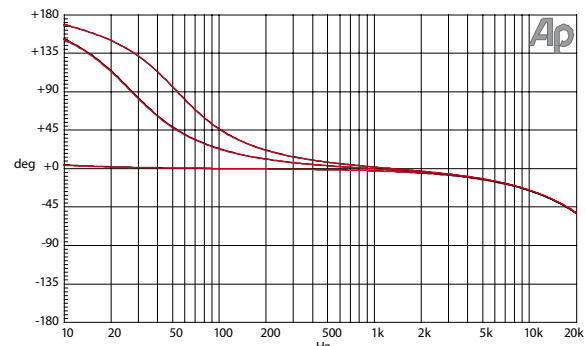
图 8.4 相位与频率 / HPF 开关的不同位置 (Ch1,Ch2) (典型性能测量值)
