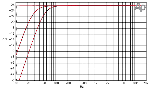
图 8.2 增益与频率 / HPF 开关的不同位置 (Ch1,Ch2) (典型性能测量值)
